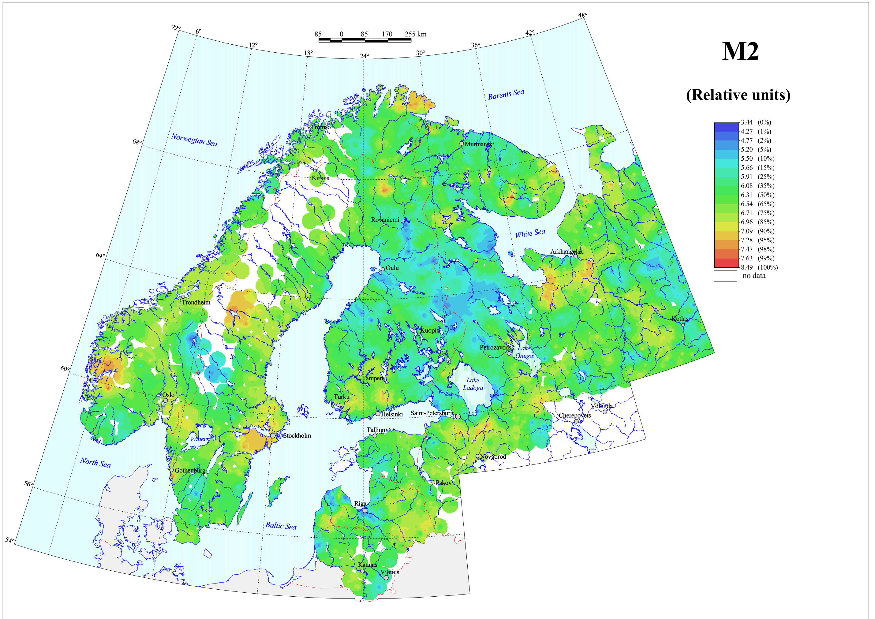
M2 (Fe, Mn) in C-horizon, Grain Size <2 mm, Aqua regia Extraction
